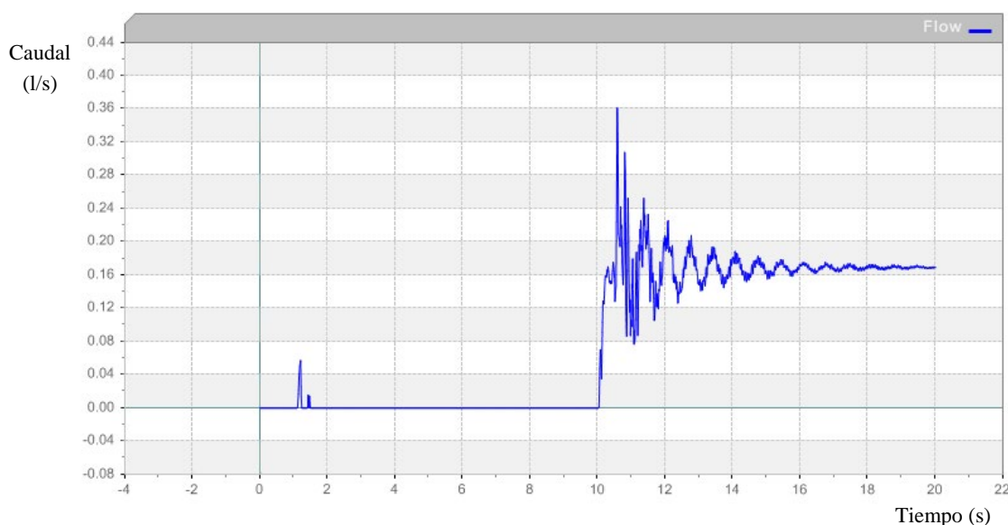
Figura 4. Caudal circulante por la tubería T20
