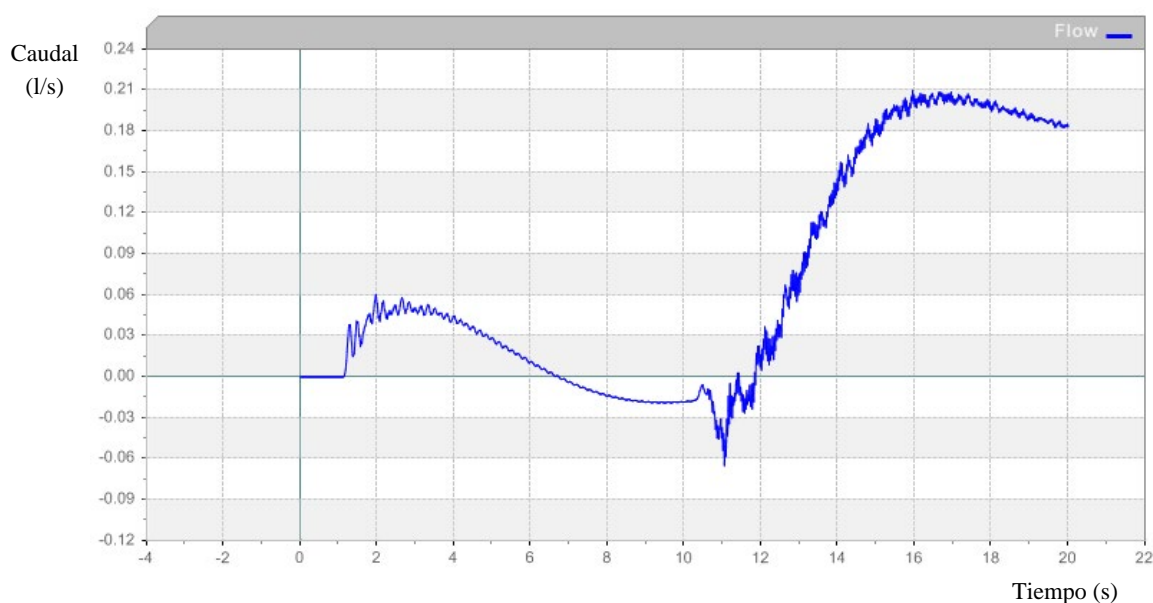
Figura 7. Caudal circulante por la montante, tubería T2
