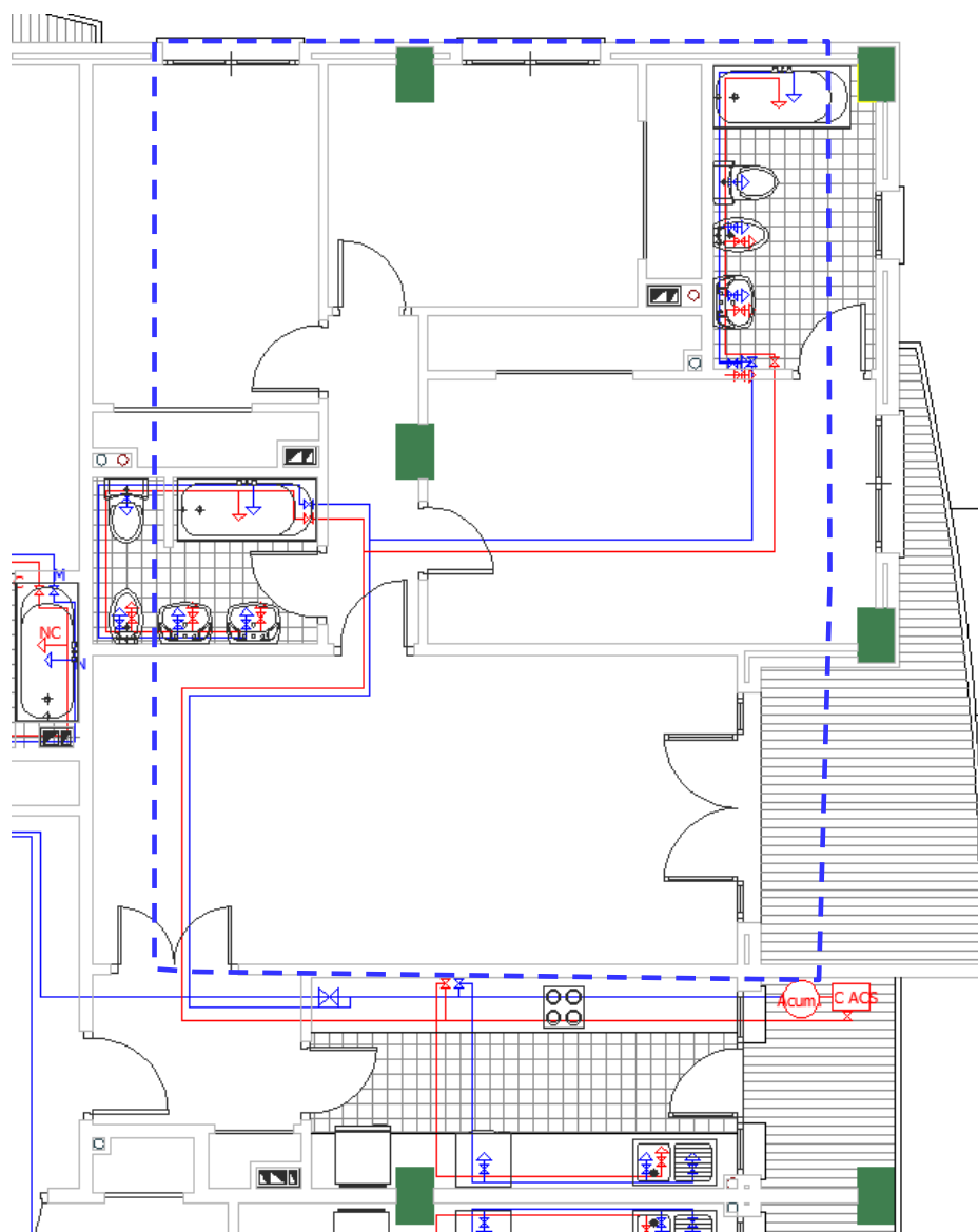
Figura 2. Instalación de la vivienda tipo considerada en el estudio.
