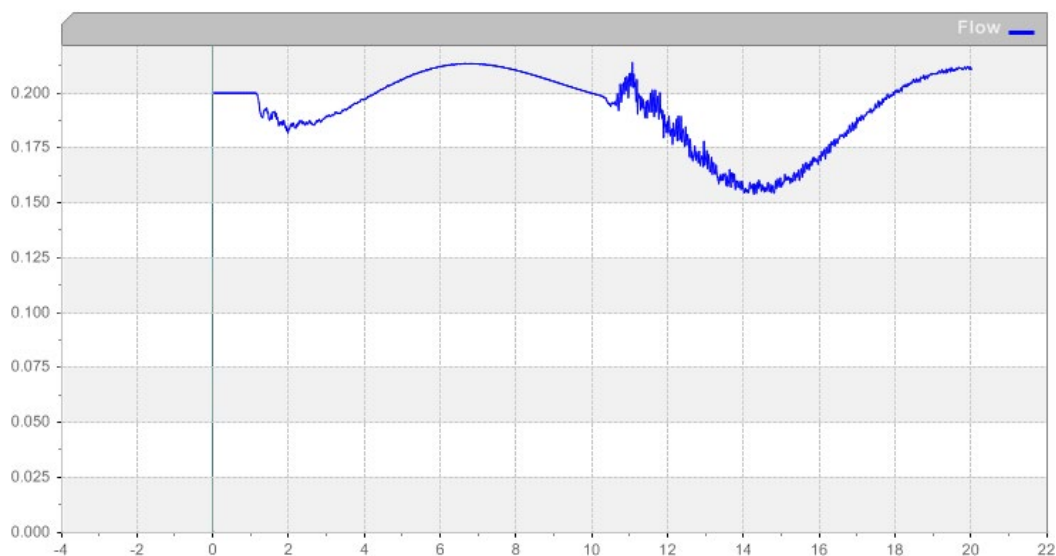
Figura 8. Caudal circulante por la tubería T8
