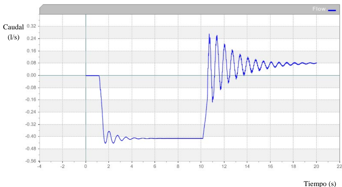
Figura 5. Caudal circulante por la tubería T13
