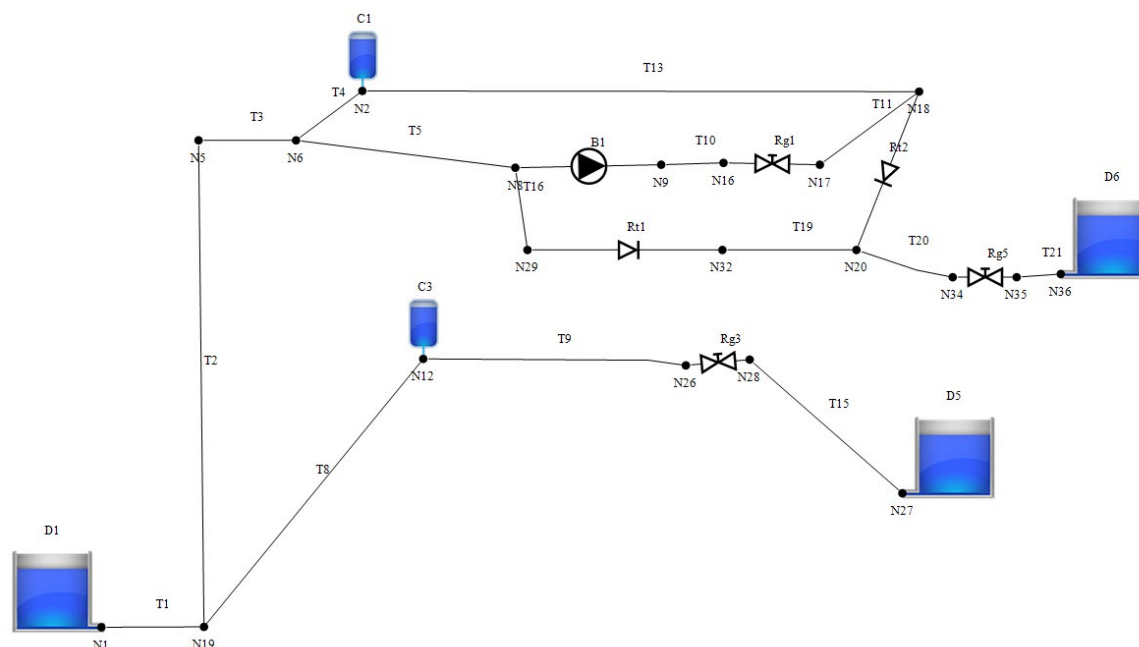
Figura 3. Esquema de la instalación utilizada para la simulación
