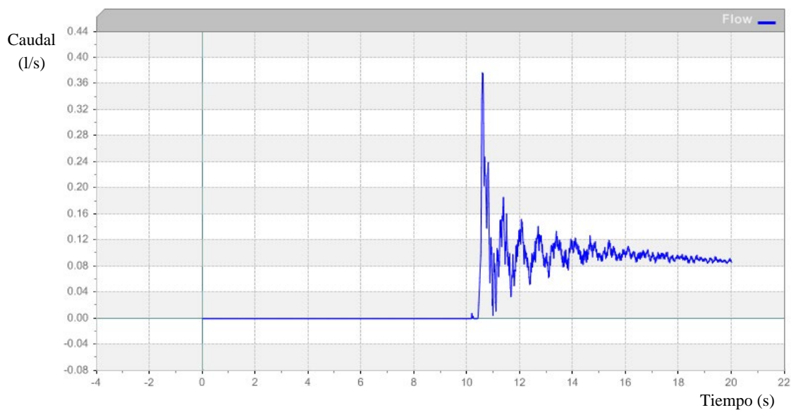
Figura 6. Caudal circulante por la tubería T19
