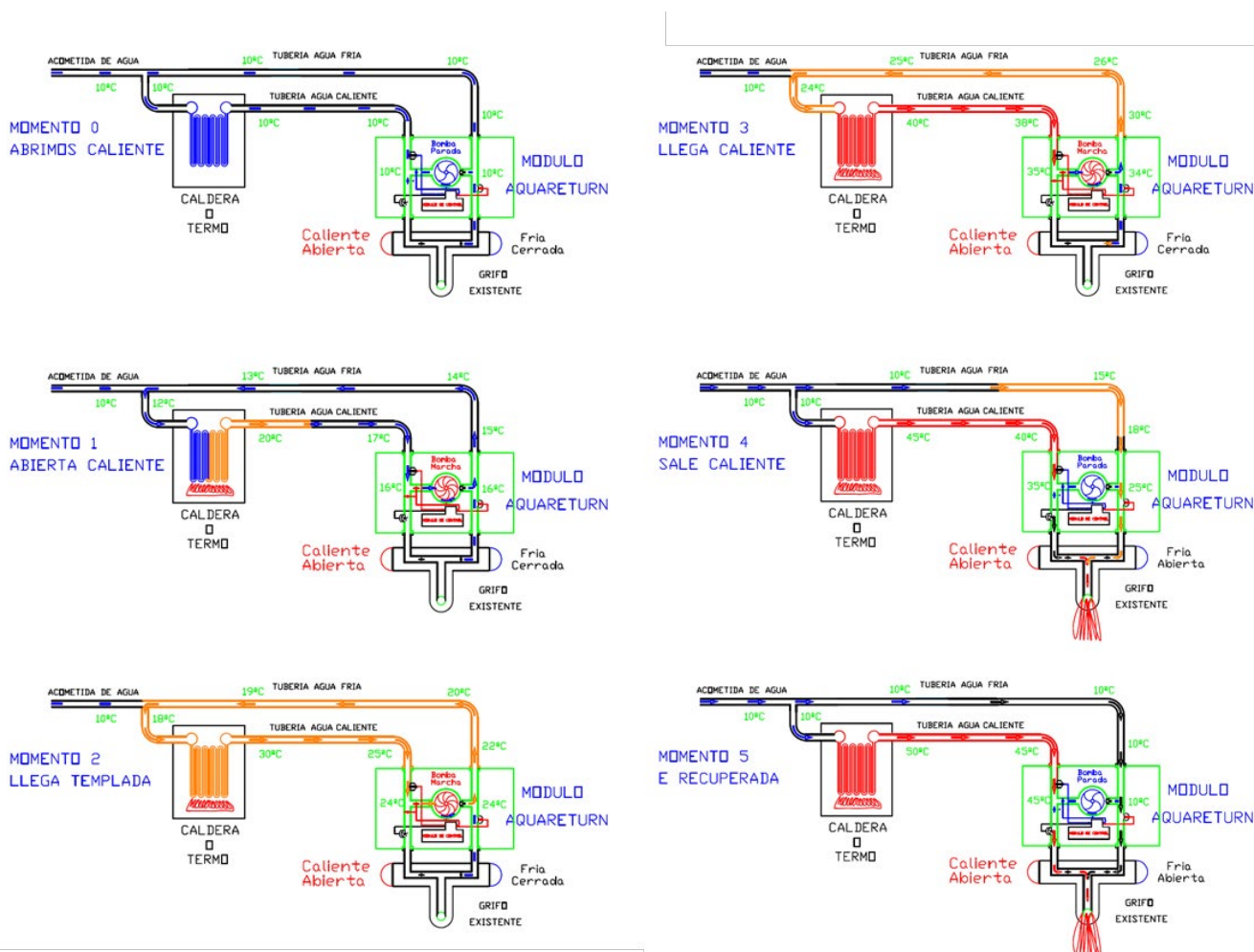
Figura 1. Fases de funcionamiento del dispositivo AQUARETURN
